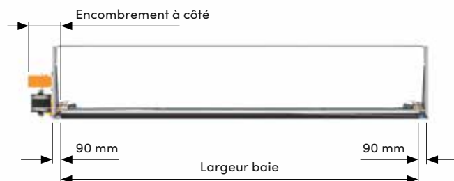
Vue de dessus du moteur à côté (standard)
