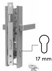
Serrure avec cylindre euro Cylindre 30/35 avec 3 clés. Poignée de porte à l'intérieur et à l'extérieur.
