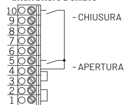
Interruttore a chiave
