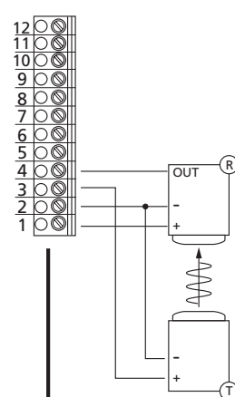
Fotocellula di transito NC, NPN, PNP
