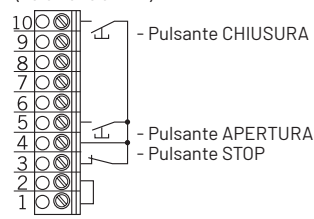
PULSANTE APERTURA / STOP / CHIUSURA (soluzione a 4 fili)
