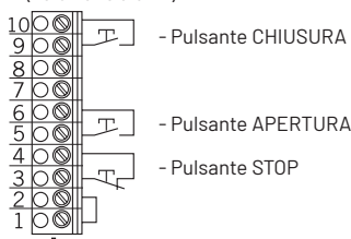
PULSANTE APERTURA / STOP / CHIUSURA (soluzione a 6 fili)
