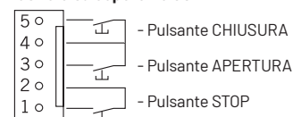
Tastiera su coperchio CS
