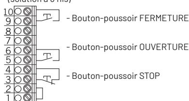
Bouton-poussoir OUVERTURE / STOP / FERMETURE (solution à 6 fils)
