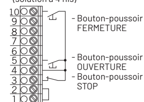
Bouton-poussoir OUVERTURE / STOP / FERMETURE (solution à 4 fils)
