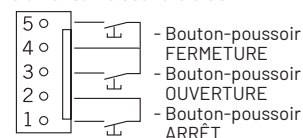
Clavier sur le couvercle CS
