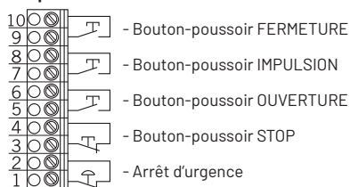
Dispositifs de commande
