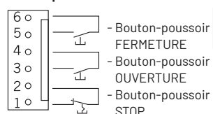
Bouton-poussoir sur le couvercle KDT
